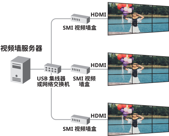
图 4：使用 SM769 为主的视频墙盒安装视频墙的架构
